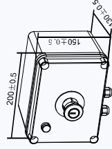
BFS-ESW21-(K)
