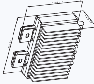
BFS-A2
