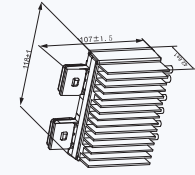
BFS-A1
